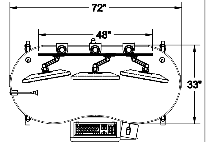
TOP VIEW SCALE: 1/2" = 1' - 0"
